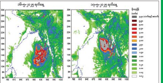
၁၂-၅-၂၀၂၅ ရက်နေ့မှ ၁၇-၅-၂၀၂၅ ရက်နေ့အတွင်း မိုးလေဝသ သင်္ချာပုံစံပြုမော်ဒယ်လ်မှ ခန့်မှန်းထားသည့် မိုးရွာသွန်းမှုအခြေအနေ ခန့်မှန်းချက်ပြပုံ။
