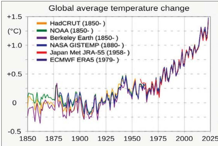
ကမ္ဘာ့ပျမ်းမျှအပူချိန် စက်မှုခေတ်မတိုင်မီကာလထက် ပိုမိုမြင့်တက်လာပုံ။
