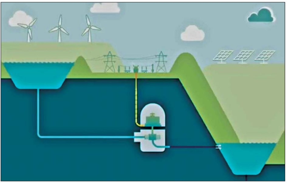
Open-loop Pumped Hydropower System အတွက် ဆိုလာနှင့် လေအား စွမ်းအင်နှစ်မျိုးဖြင့် ရေတင်မှု သရုပ်ပြပုံ။
