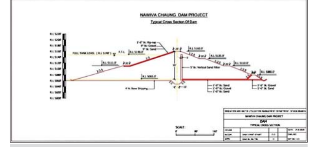
နွယ်ချောင်းဆည်ရေလှောင်တံ တည်ဆောက်မည့် ဒီဇိုင်းပုံစံ။ ရေလှောင်တံကို တည်ဆောက်မည့် လိုအပ်လျက်ရှိသော သောက်သုံးရေ ဖြစ်ပြီး ဆည်တည်ဆောက်ပြီးပါက ဒေသခံပြည်သူများအတွက် နေ့စဉ် လိုအပ်လျက်ရှိသော သောက်သုံးရေ ဖြစ်ပေးနိုင်မည်ဖြစ်ကြောင်း သိရ သည်။ ခရိုင်(ပြန်/ဆက်)
