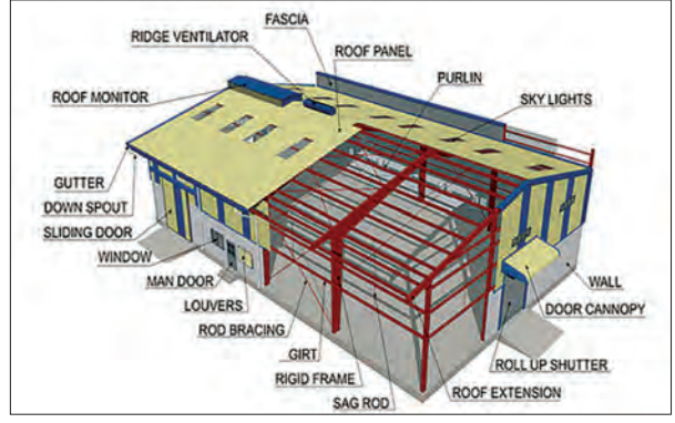
အဆောက်အအုံတစ်ခုတွင် လေမုန်တိုင်းဒဏ်ကာကွယ်နိုင်ရန် လေဝင်လေထွက်ပေါက်များ ထားရှိပုံ
