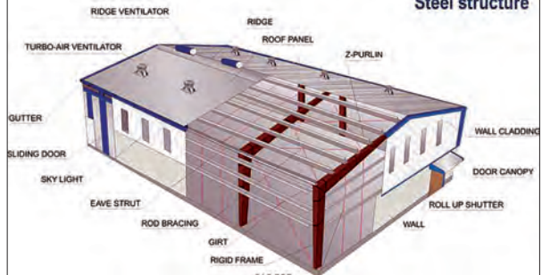
Steel Structure ပုံစံပြထားမှုကို တွေ့ရစဉ်
