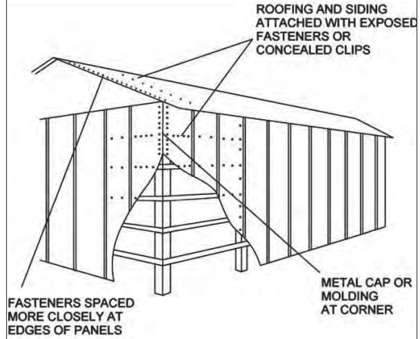
သစ်သားအဆောက်အအုံအား မူလီ၊ သံမိုတို့စိပ်စိပ်ထည့်၍ မုန်တိုင်းဒဏ်ခံအောင် တည်ဆောက်ထားပုံ
