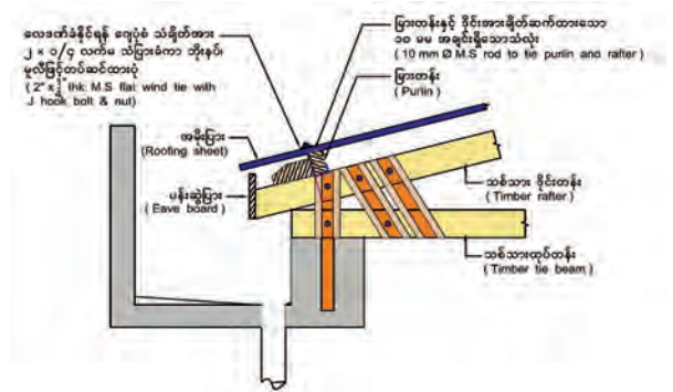
အဆောက်အအုံများတွင် အမိုးများလေမလှန်နိုင်အောင် တည်ဆောက်ထားမှုကို တွေ့ရစဉ်
