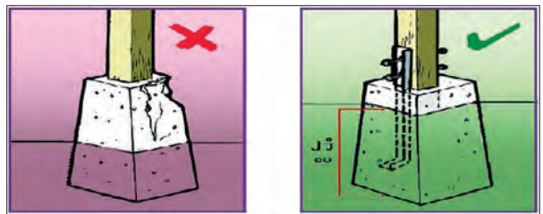
ကွန်ကရစ်ဖိနပ်တိုင်ခံတည်ဆောက်ပုံအမှားအမှန်ကို တွေ့ရစဉ်
