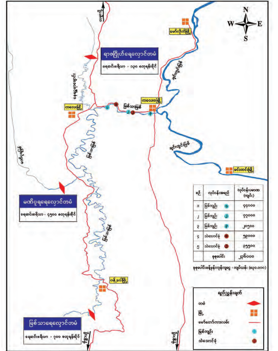
မြစ်သာမြစ်ကျဉ်းများ ချဲ့ထွင်တူးဖော်ခြင်းလုပ်ငန်း မြစ်သာမြစ်ပေါ်ရှိ ချဲ့ထွင်တူးဖော်ရမည့် မြစ်ကျဉ်း (၃)ခုနှင့် သဲသောင်ခုံ (၂) ခု တည်နေရာပြပုံ
