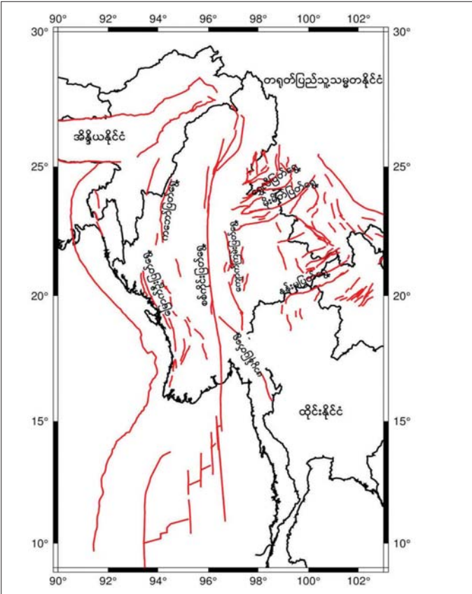
မြန်မာနိုင်ငံတွင် ငလျင်လှုပ်ရှားမှုဖြစ်ပေါ်စေသော ပြတ်ရွေ့များပြပုံ။
