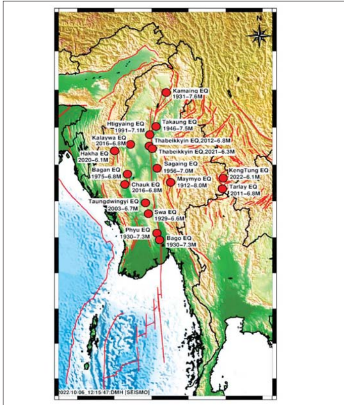
မြန်မာနိုင်ငံတွင် လှုပ်ရှားခဲ့သော သမိုင်းဝင် အင်အားပြင်းငလျင်များ၏ မြေပြင်ဗဟိုချက်များပြပုံ။
