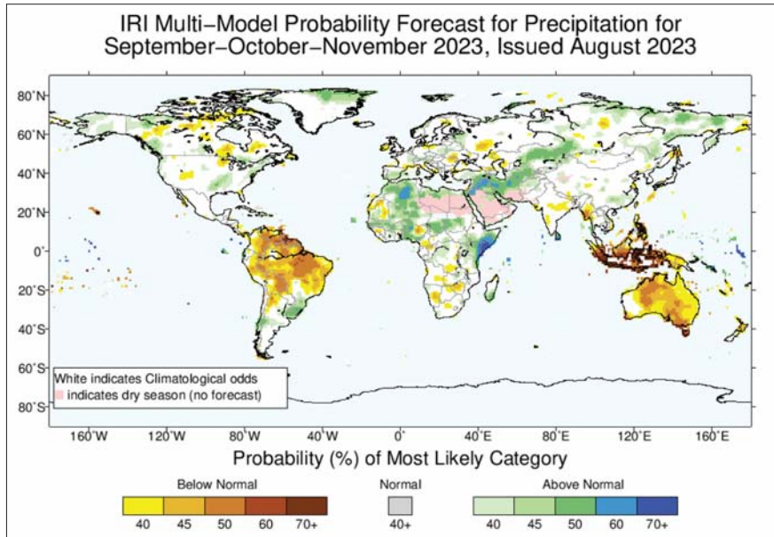
ပုံ(၂)၂၀၂၃ခုနှစ် စက်တင်ဘာ၊ အောက်တိုဘာနှင့် နိုဝင်ဘာလများအတွင်း ကမ္ဘာတစ်ဝန်း မိုးရွာသွန်းမှုအခြေအနေခန့်မှန်းချက်မြေပုံ (သတင်းရင်းမြစ်-အပြည်ပြည်ဆိုင်ရာ ရာသီဥတုနှင့် လူထုဆိုင်ရာ သုတေသနဌာန(IRI))
