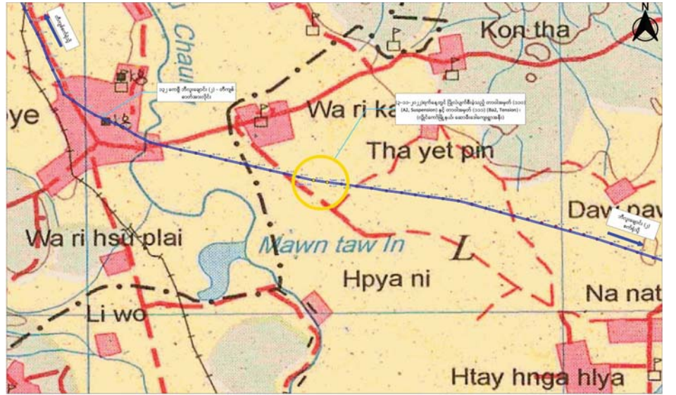
၁၃၂ ကေစီ ဘီလူးချောင်း(၂)-တီကျပ် နှစ်ထပ်ဓာတ်အားလိုင်း တာဝါတိုင်အမှတ်(၁၁၀)နှင့် (၁၁၁) ဖောက်ခွဲဖျက်ဆီးခံရသည့် တည်နေရာပြမြေပုံ။
