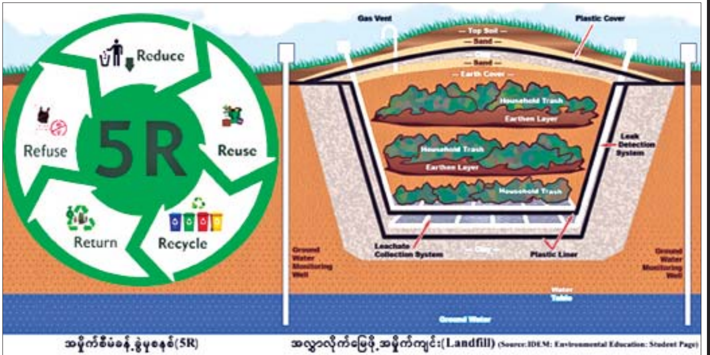
အမှိုက်စီမံခန့်ခွဲမှုစနစ်နှင့် အလွှာလိုက်မြေဖို့အမှိုက်ကျင်းဖြတ်ပိုင်းပုံ။
