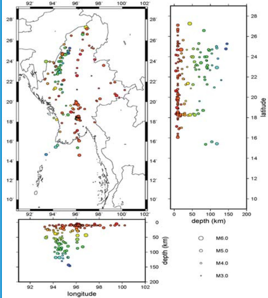
၂၀၁၈ ခုနှစ်အတွင်း သတင်းထုတ်ပြန်ခဲ့သော မြေငလျင်လှုပ်ရှားမှုများ၏ cross section ဖြင့် ရေးဆွဲထားသော မြေပုံ
