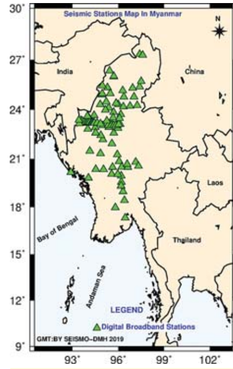
ယာယီမြေငလျင်စခန်း (၉၀) တပ်ဆင်ထားရှိမှုပြမြေပုံ
