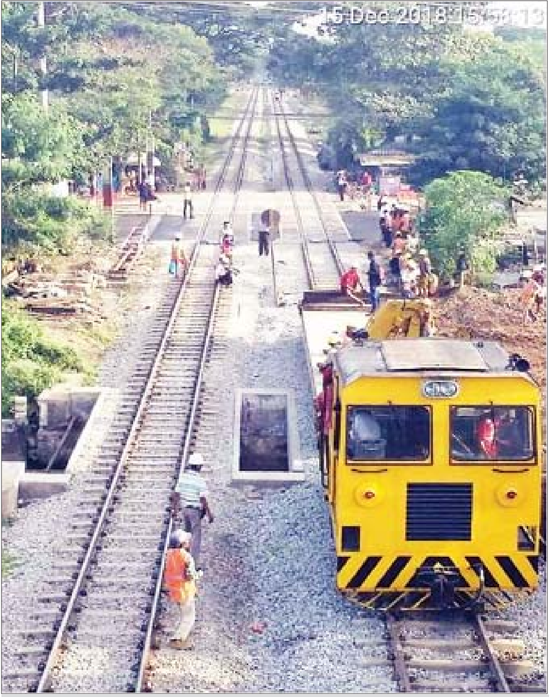
ရထားလမ်းအဆင့်မြှင့်တင်ရေးလုပ်ငန်းဆောင်ရွက်နေမှုကို တွေ့ရစဉ်။
