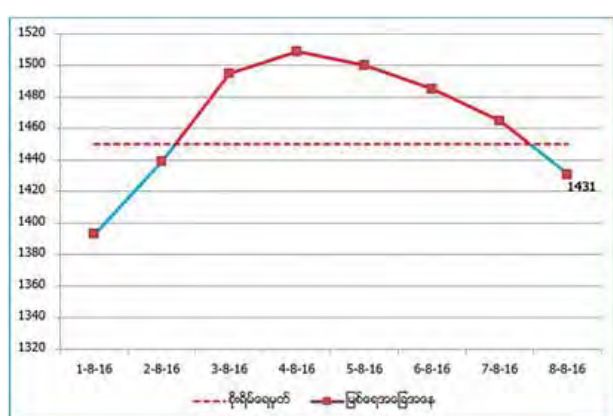
ချောက်မြို့၊ ဧရာဝတီမြစ်ဝကျွန်းပေါ်ရေအဆင့် (စင်တီမီတာ)
