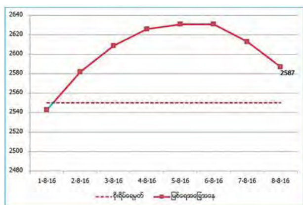
အောင်လံမြို့၊ ဧရာဝတီမြစ်ဝကျွန်းပေါ်ရေအဆင့် (စင်တီမီတာ)
