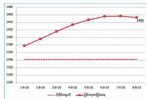
ဟင်္သာတမြို့၊ ဧရာဝတီမြစ်ဝကျွန်းပေါ်ရေအဆင့် (စင်တီမီတာ)
