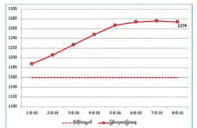
ညောင်ဦးမြို့၊ ဧရာဝတီမြစ်ဝကျွန်းပေါ်ရေအဆင့် (စင်တီမီတာ)
