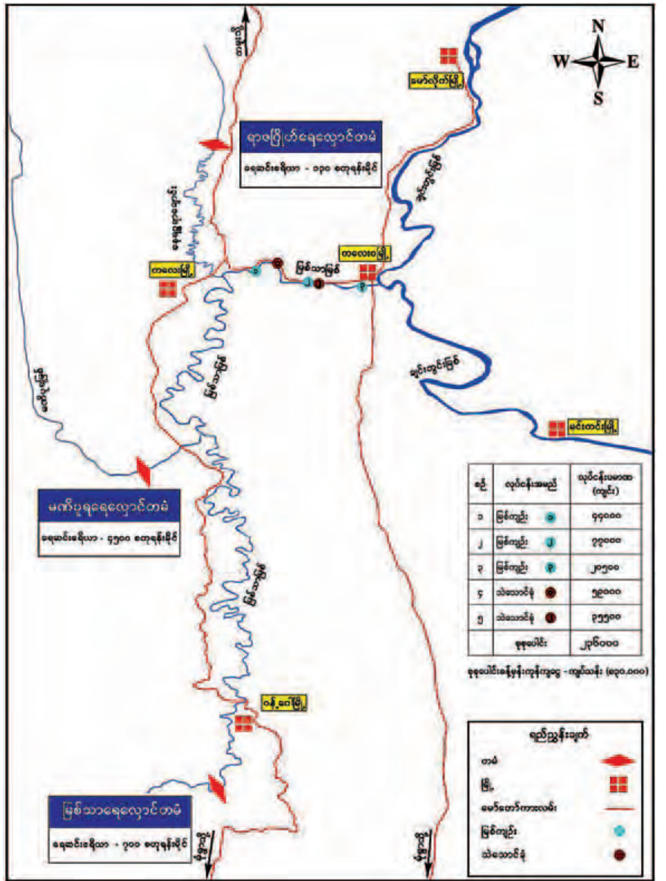
မြစ်သာမြစ်ကျဉ်းများ ချဲ့ထွင်တူးဖော်ခြင်းလုပ်ငန်း မြစ်သာမြစ်ပေါ်ရှိ ချဲ့ထွင်တူးဖော်ရမည့် မြစ်ကျဉ်း သုံးခုနှင့် သဲသောင်ခုံ နှစ်ခု တည်နေရာပြပုံ။
