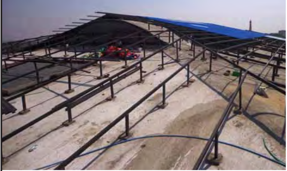
လိုဏ်ဂူတော်အစိုးရအဖွဲ့ Hollow Pipe ဖရိန်များဖြင့် ပြန်လည်မွမ်းမံ ပြင်ဆင်နေစဉ်။
