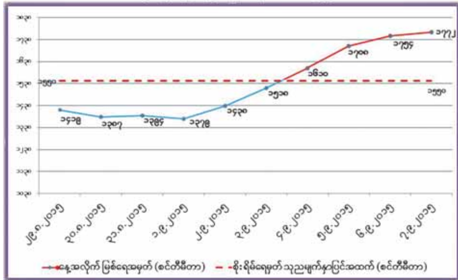
ချင်းတွင်းမြစ်ရေ အခြေအနေ (ကလေးမြို့)
