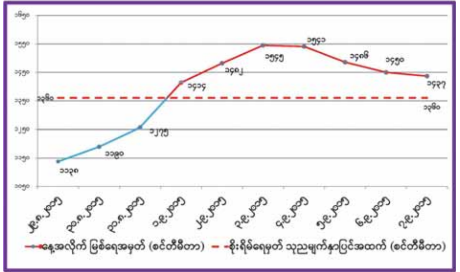
ချင်းတွင်းမြစ်ရေ အခြေအနေ (မော်လိုက်မြို့)
