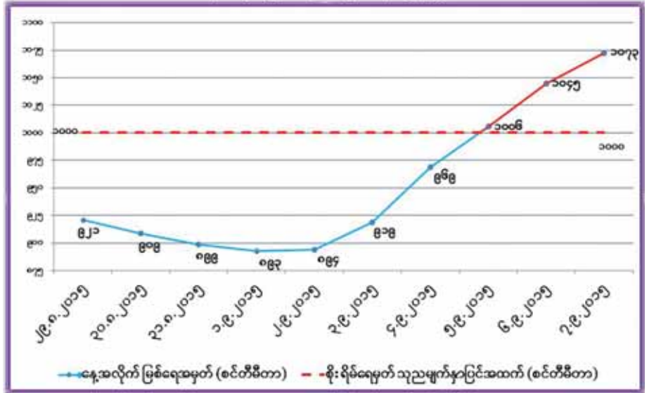
ချင်းတွင်းမြစ်ရေ အခြေအနေ (မုံရွာမြို့)
